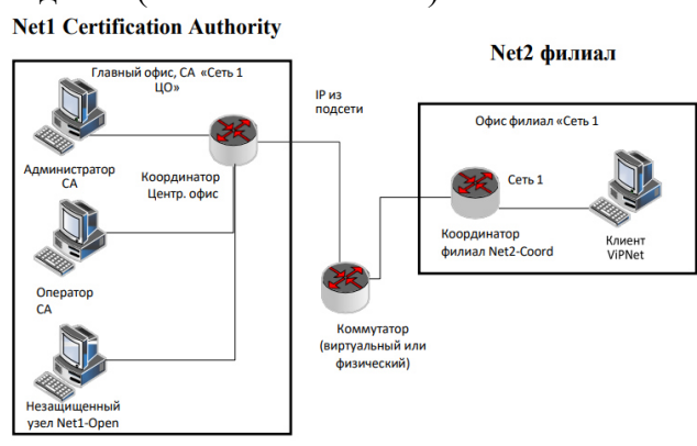
Рисунок 1 Схема защищенной сети
