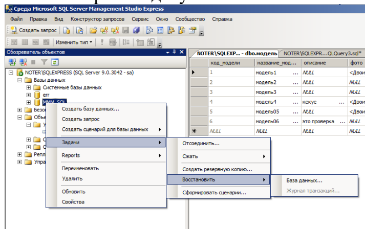
Рисунок 6 – Восстановление БД
