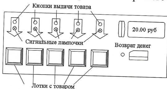
Рис. 4.2. Лицевая панель торгового автомата
