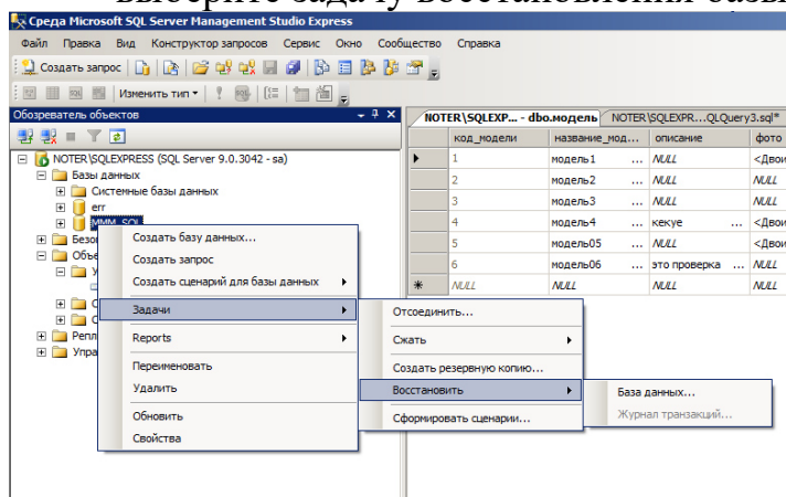
Рисунок 6 – Восстановление БД
